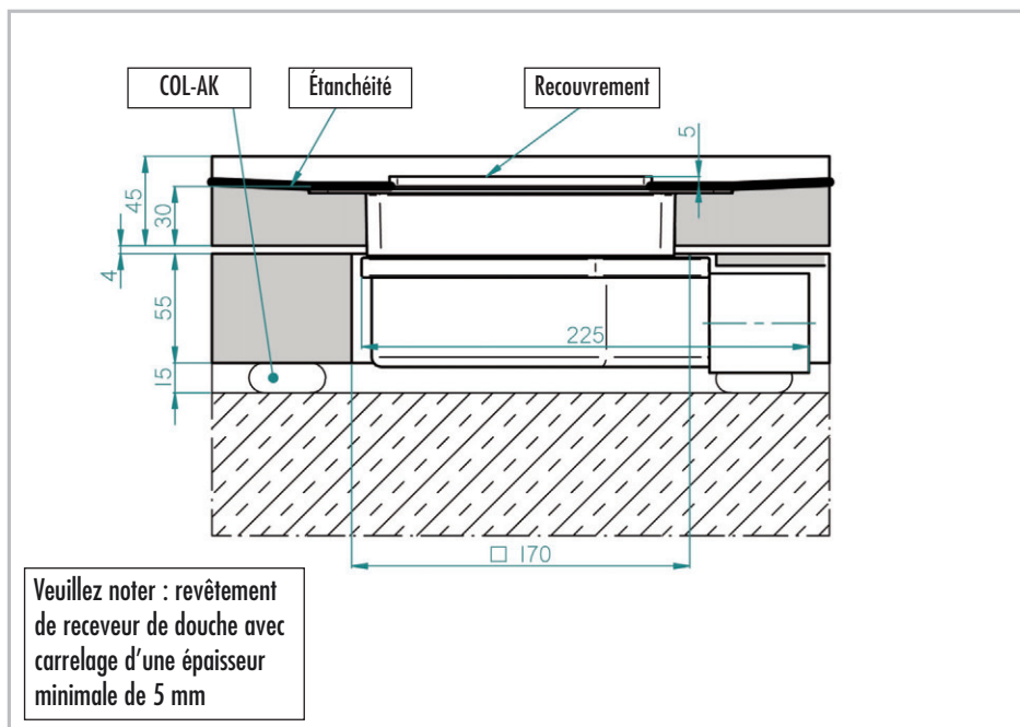
– Siphon de sol horizontale avec obturateurs d'odeurs amovible, DN 50
