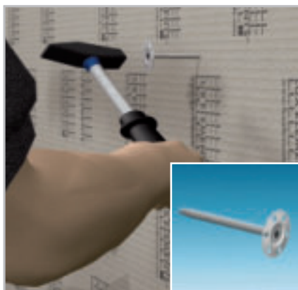
FIX-FID – Cheville à frapper
