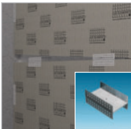
MONT-H – Assemblage d'éléments porteurs en mousse dure
