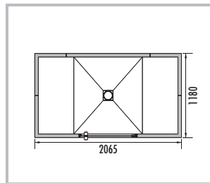
■ MODUL-CAB-R 2065/1180 rectangulaire, 2 x banquette de forme SOLO
