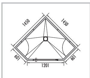
■ MODUL-CAB-F 1450 pentagonal, 2 x banquette de forme SOLO en quart de cercles
