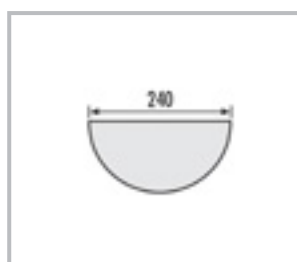
■ DECO-PM H Pilier, semi rond, ∅ 240 mm, longueur 2500 mm
