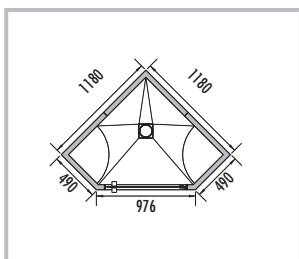
■ MODUL-CAB-F 1180 pentagonal, 2 x banquette de forme SOLO en quart de cercles
