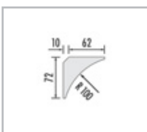
■ DECO-HK 100 Élément en forme de gorge, longueur 2500 mm
