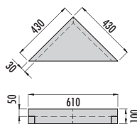
■ RELAX-BA-CO FLOAT S Banquette suspendue de forme triangulaire CORNER FLOAT S, inclus kit de montage, composé de : 6 pièces FIX-SB 80S35, 4 pièces FIX-SD 80, 1 cartouche COL-MK
