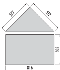
■ RELAX-BA-CO Banquette de forme CORNER, triangulaire
