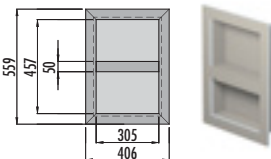
■ RELAX-NI-L avec 1 étagère, livrée séparément
