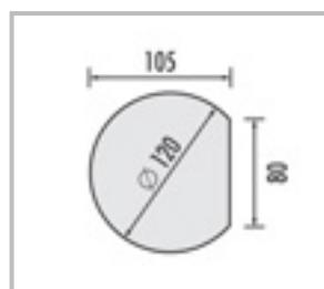
■ DECO-AE Élément de finition pour bord, Ø 120 mm, longueur 2500 mm
