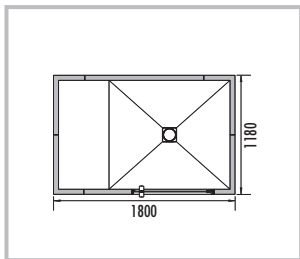
■ MODUL-CAB-R 1800/1180 rectangulaire, 1 x banquette de forme SOLO
