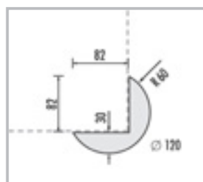
■ DECO-VE 120 Élément d'habillage rond pour les angles, Ø 120 mm, longueur 2500 mm
