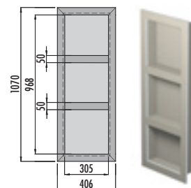
■ RELAX-NI-XL avec 2 étagères, livrées séparément
