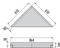
■ RELAX-BA-CO FLOAT L Banquette suspendue de forme triangulaire CORNER FLOAT L, inclus kit de montage, composé de : 6 pièces FIX-SB 80S35, 4 pièces FIX-SD 80, 1 cartouche COL-MK
