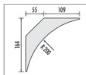
■ DECO-HK 200 Élément en forme de gorge, longueur 2500 mm
