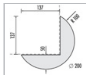
■ DECO-VE 200 Élément d'habillage rond pour les angles, Ø 200 mm, longueur 2500 mm
